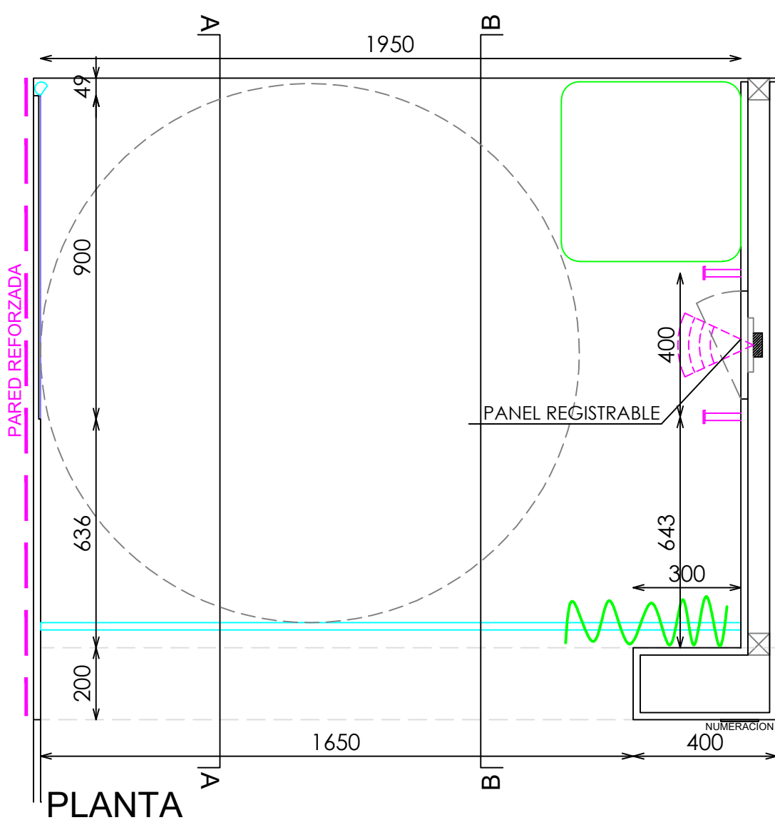
PLANTA
