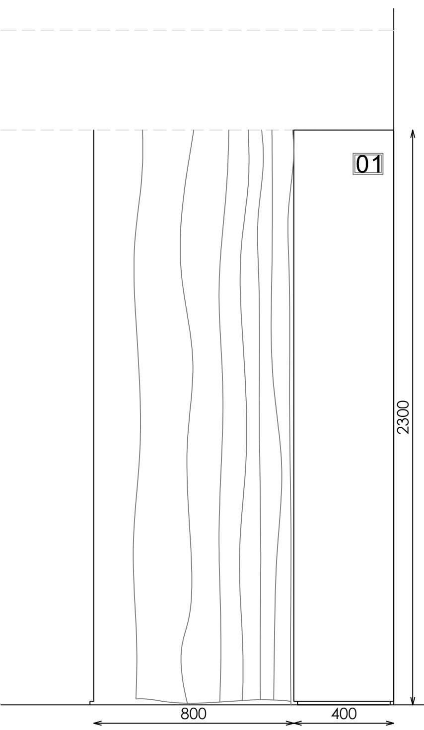
ALZADO
