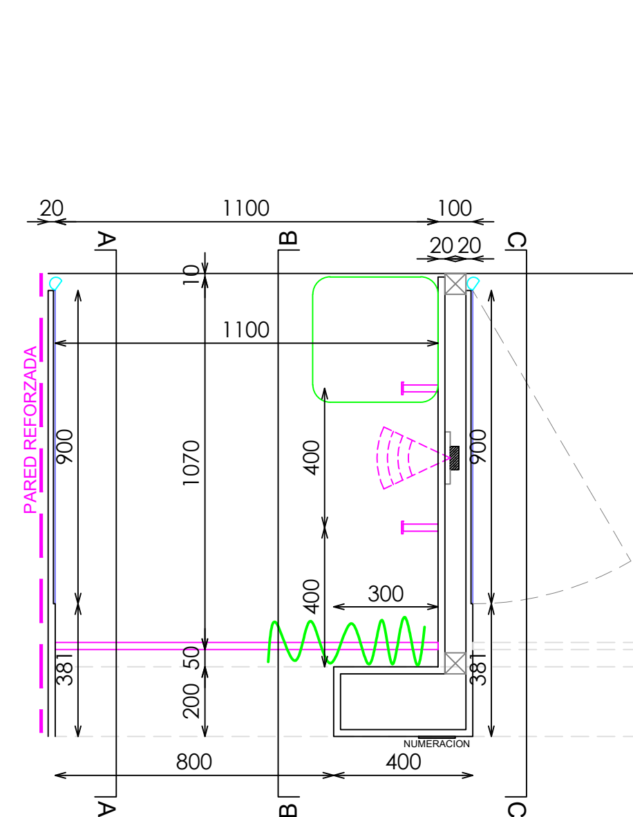
PLANTA
