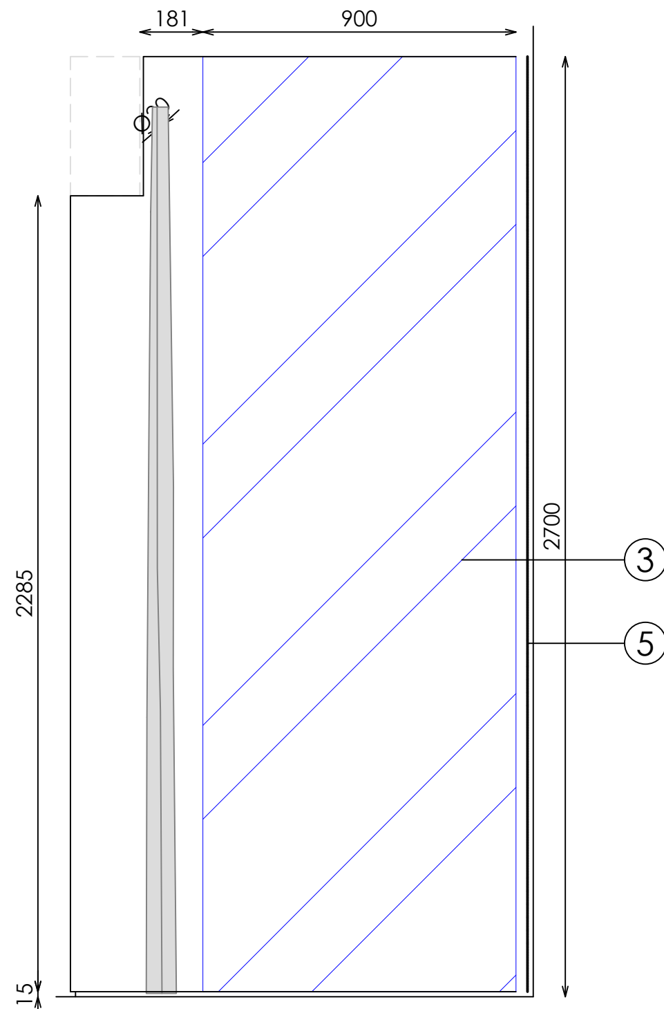
ALZADO LATERAL ESPEJO (A-A)
