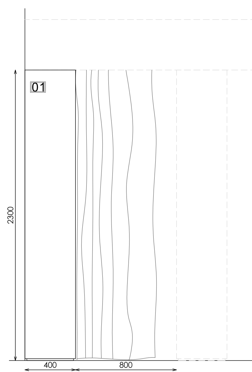
ALZADO
