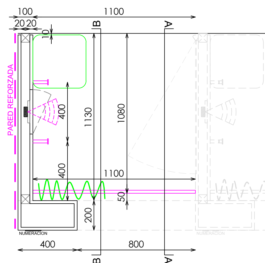
PLANTA
