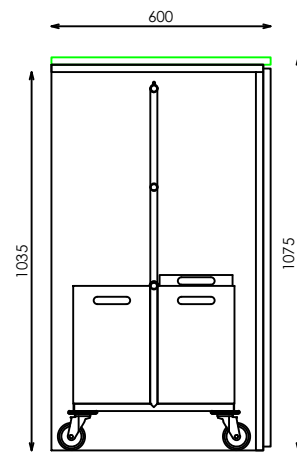
SECCION
