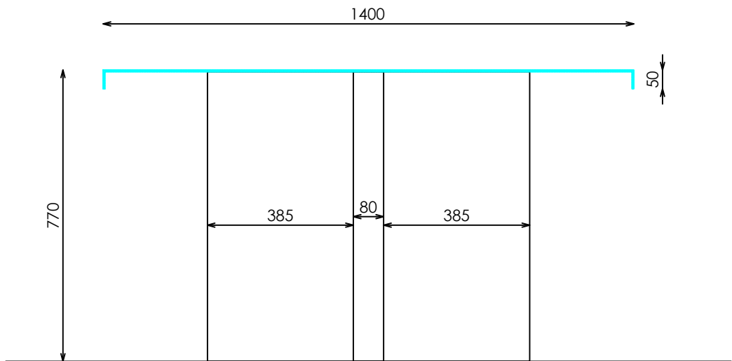
ALZADO LATERAL
