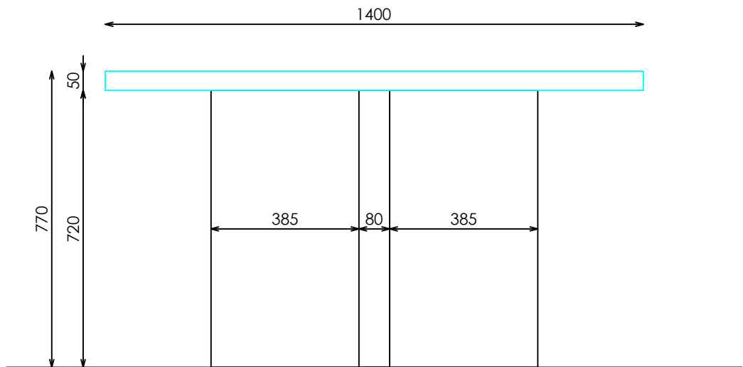
ALZADO FRONTAL
