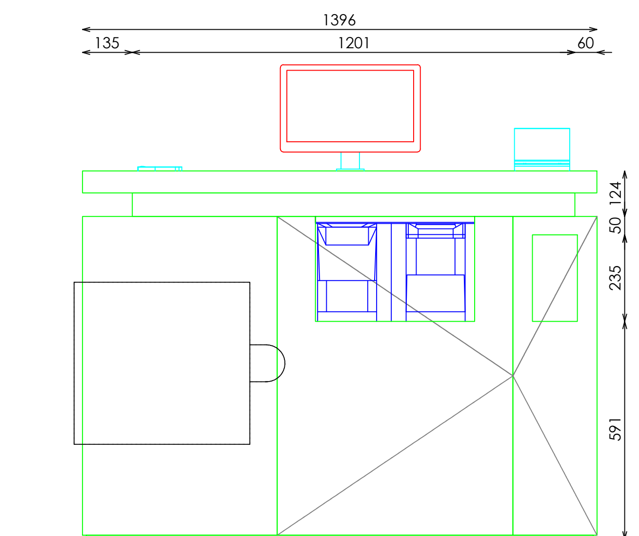
ALZADO TRASERO
