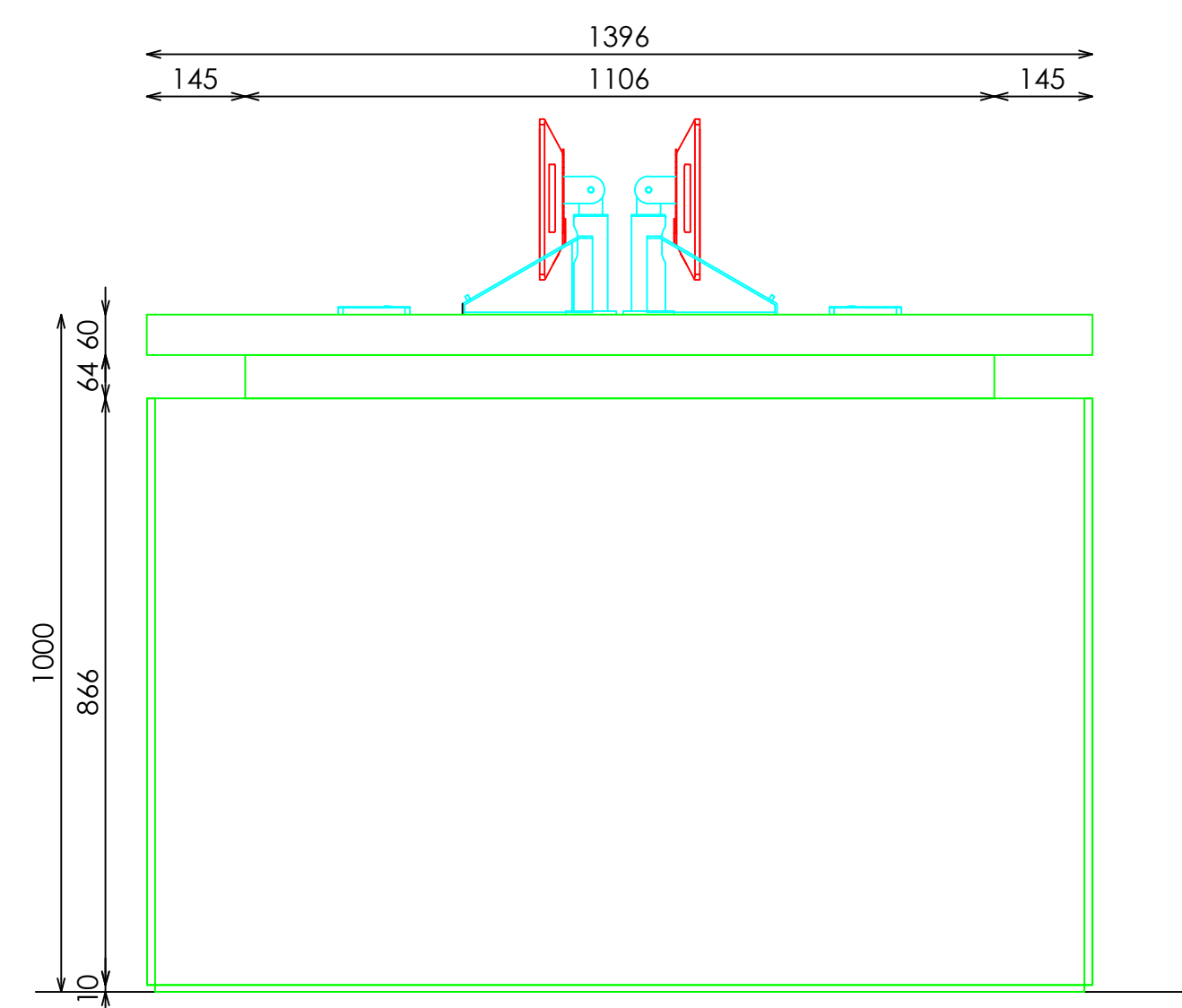
ALZADO IZQUIERDO
