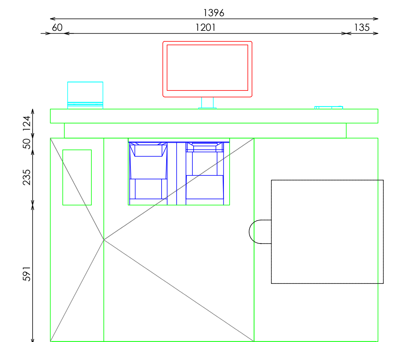
ALZADO FRONTAL
