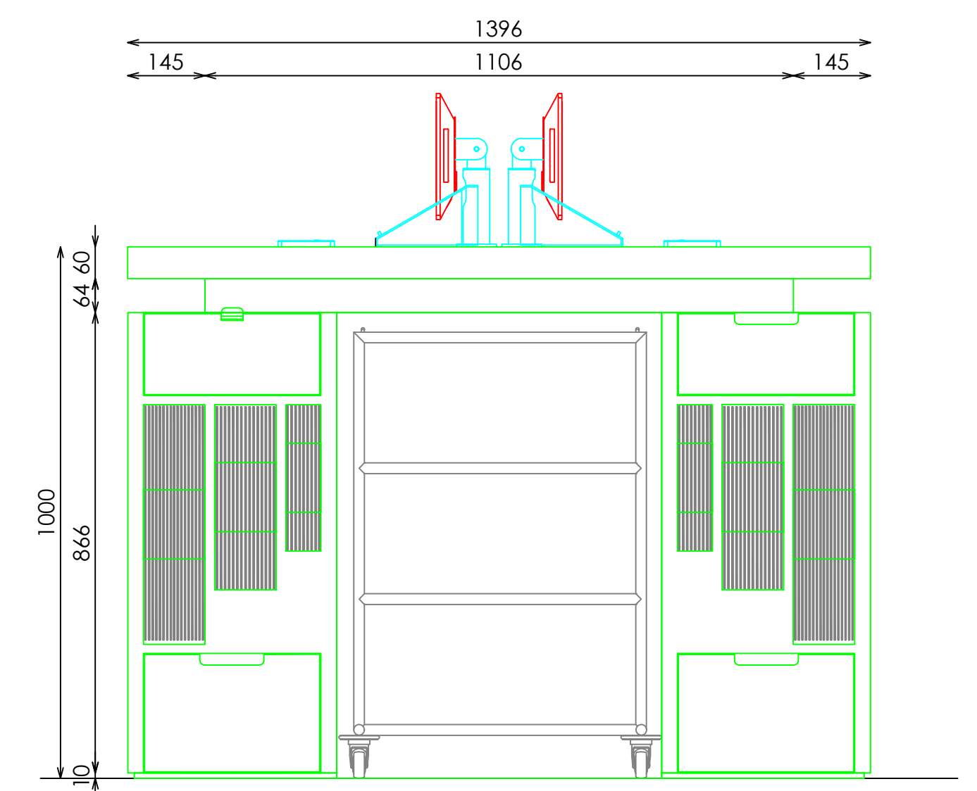
ALZADO DERECHO
