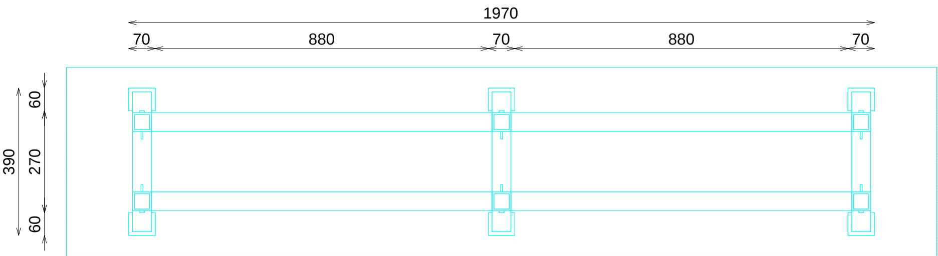
PLANTA SECCIONADA
