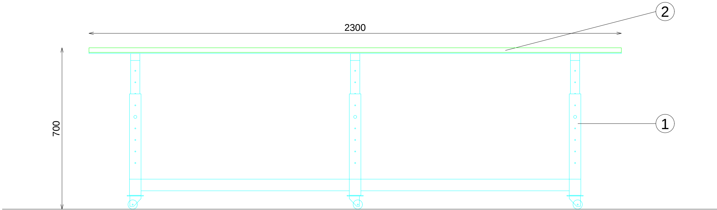
ALZADO
