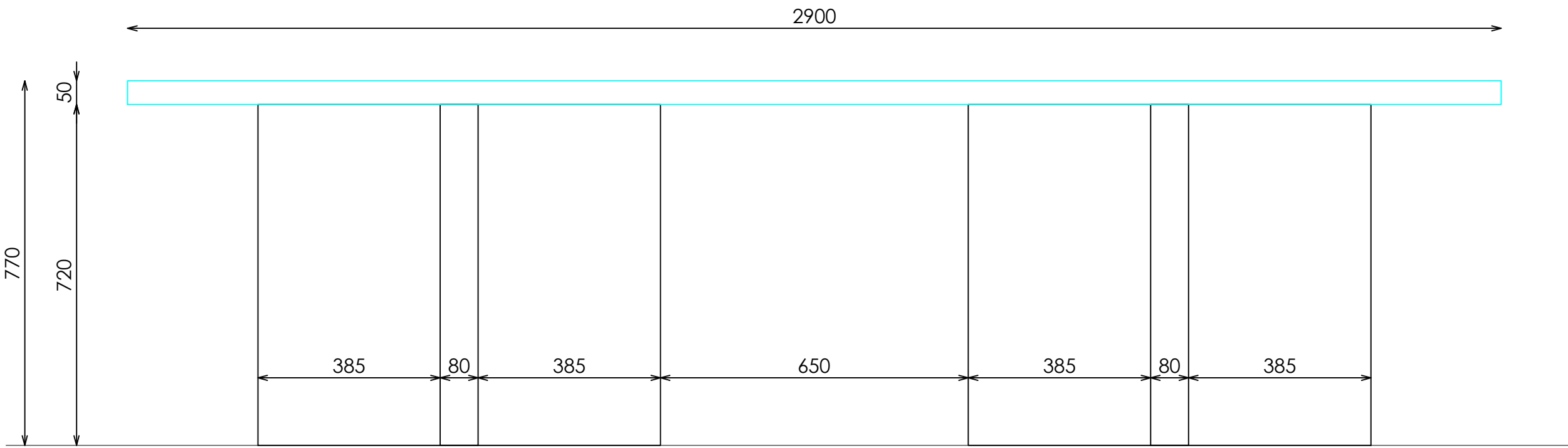
ALZADO FRONTAL
