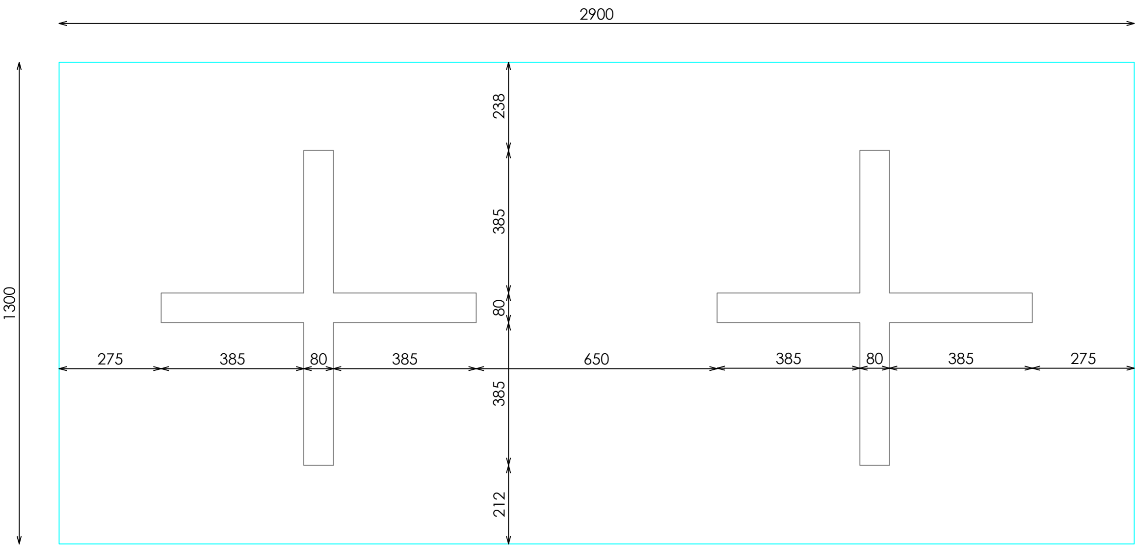
PLANTA
