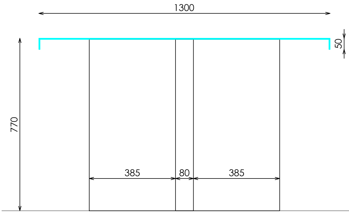
ALZADO LATERAL
