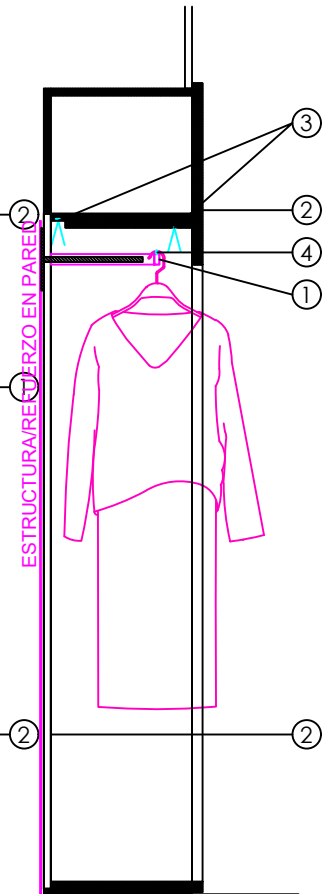
SECCIÓN BARRA ALTA
