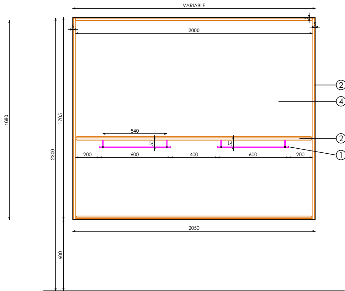
ALZADO FRONTAL
