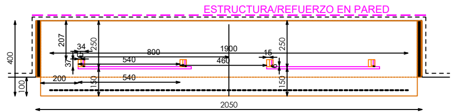
PLANTA
