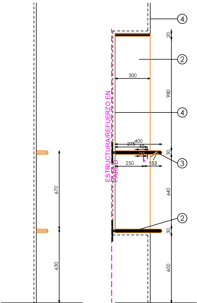
ALZADO LATERAL
