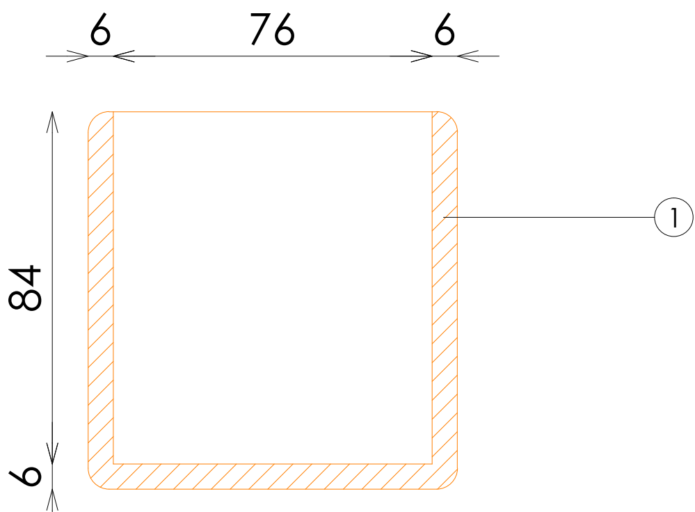
PERFIL SECCIONADO
