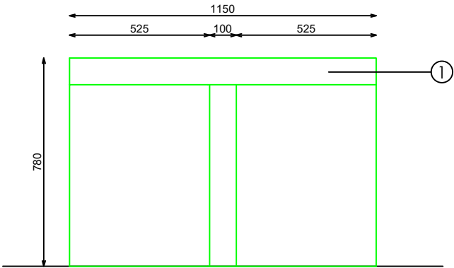
ALZADO LATERAL
