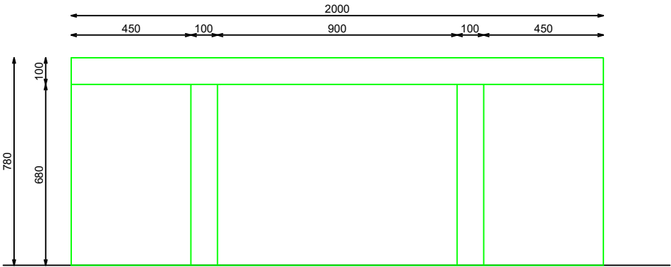
ALZADO FRONTAL
