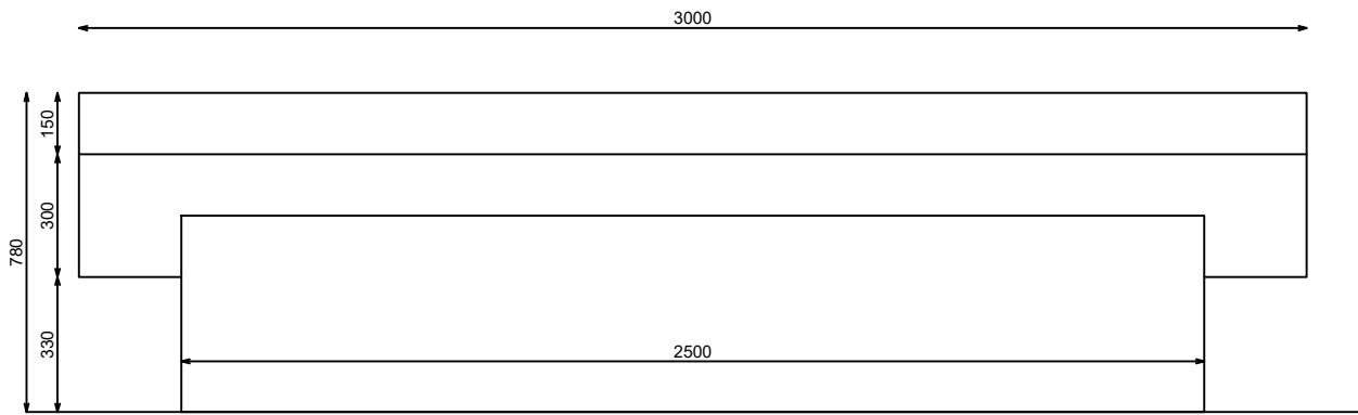
ALZADO LATERAL
