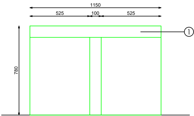
ALZADO LATERAL
