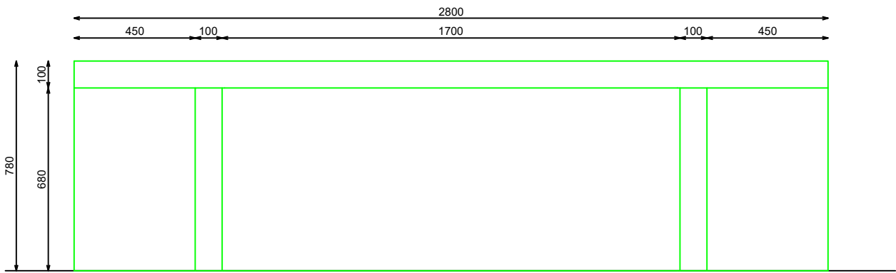
ALZADO FRONTAL
