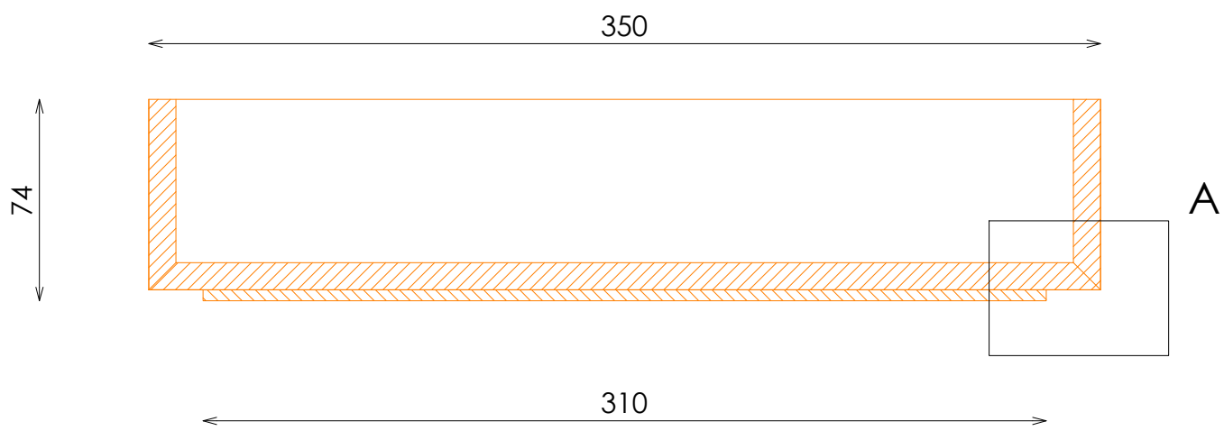
SECCION
