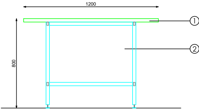
ALZADO LATERAL
