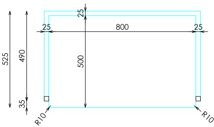
PLANTA
