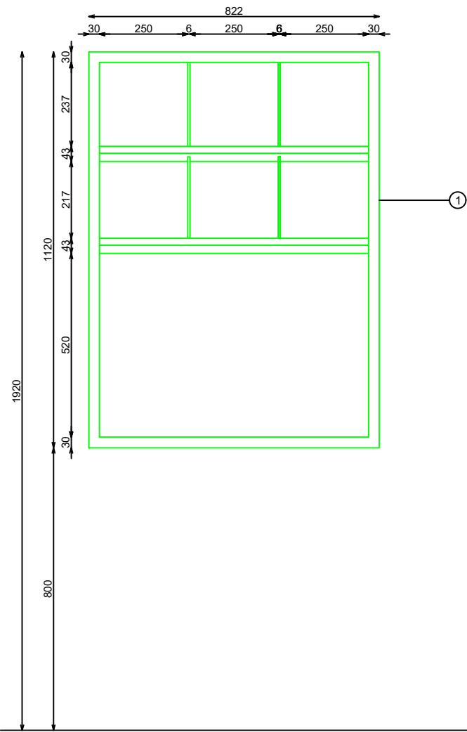
ALZADO
