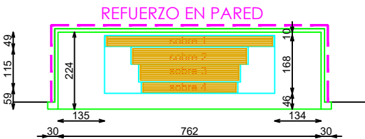
PLANTA DISTRIBUCIÓN
