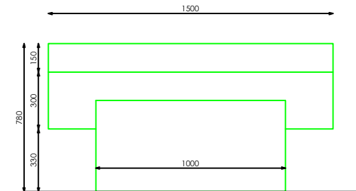
ALZADO LATERAL
