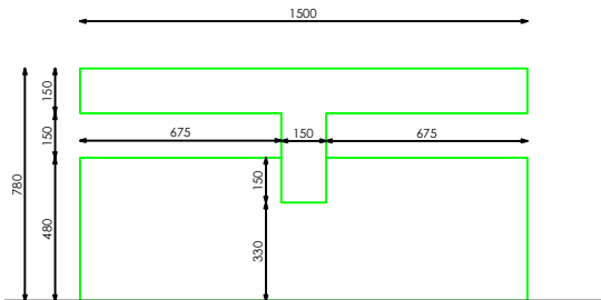
ALZADO FRONTAL
