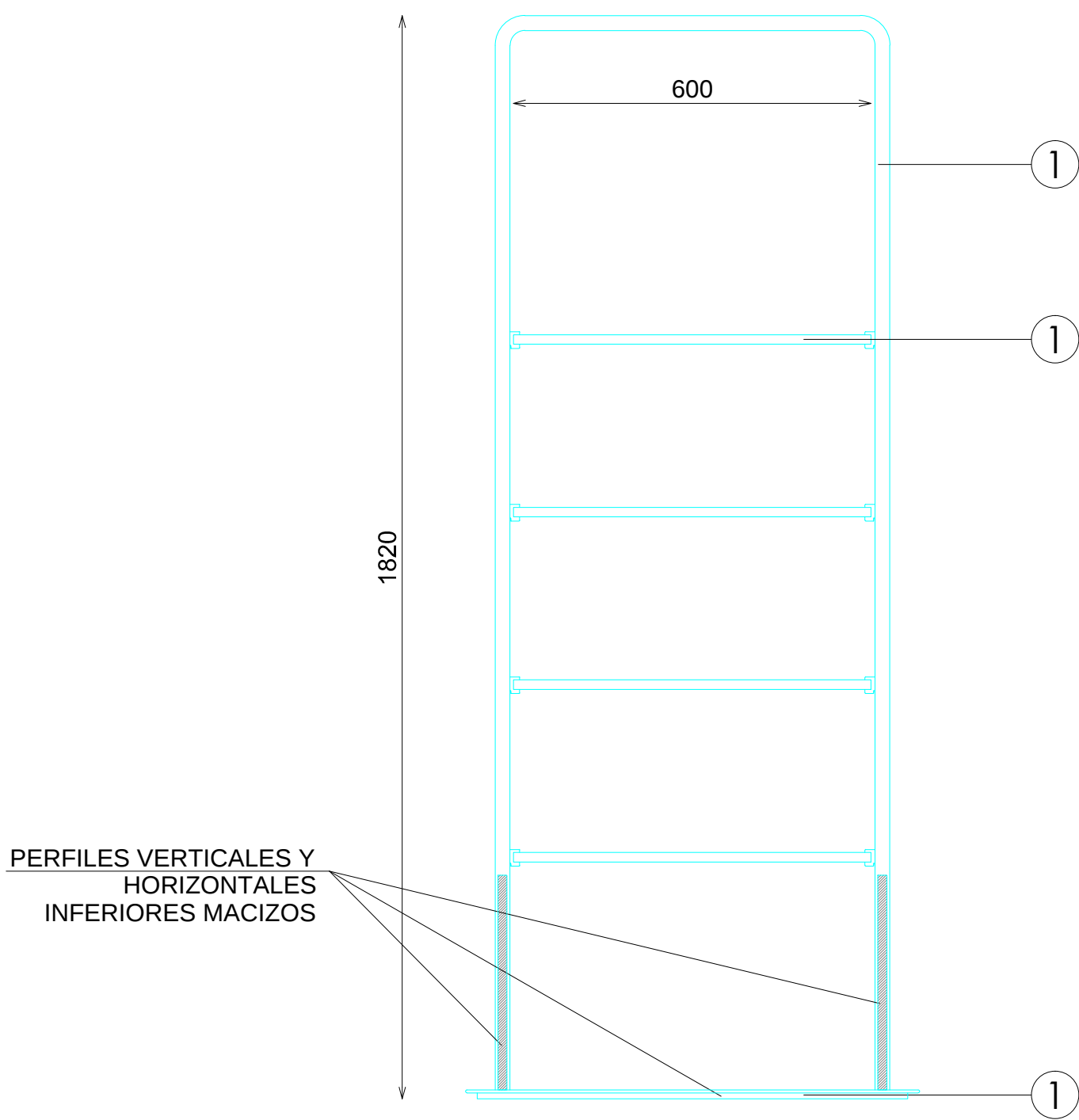
ALZADO
