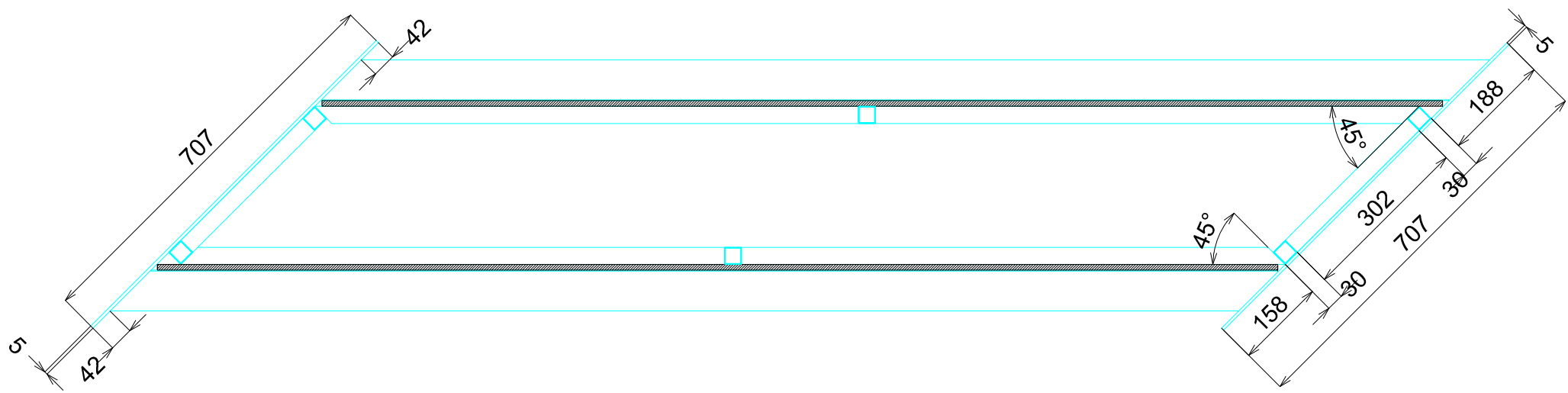
PLANTA EN SECCION
