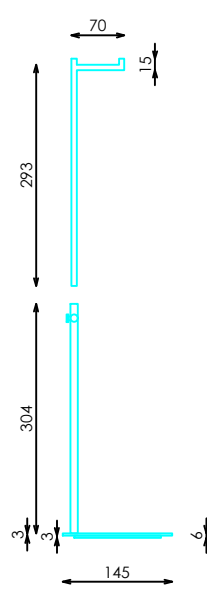
ALZADO D
