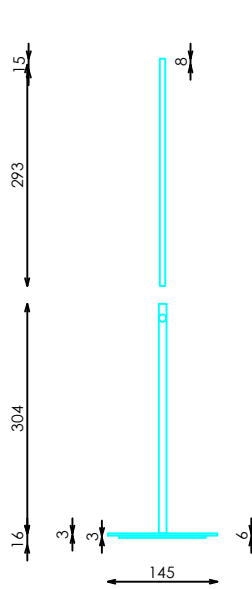
ALZADO C
