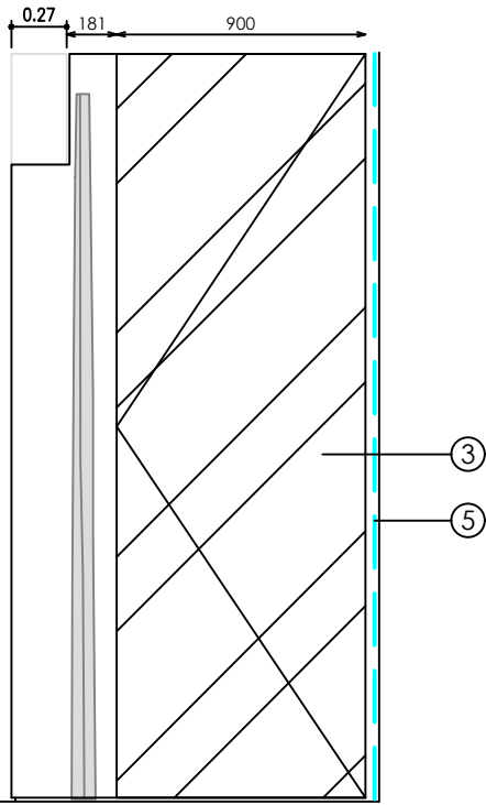
ALZADO LATERAL ESPEJO (A-A)
