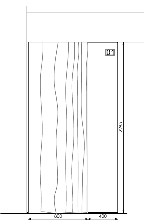
ALZADO
