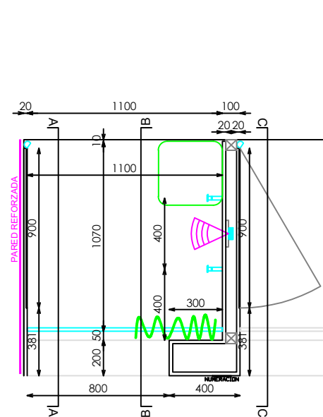
PLANTA
