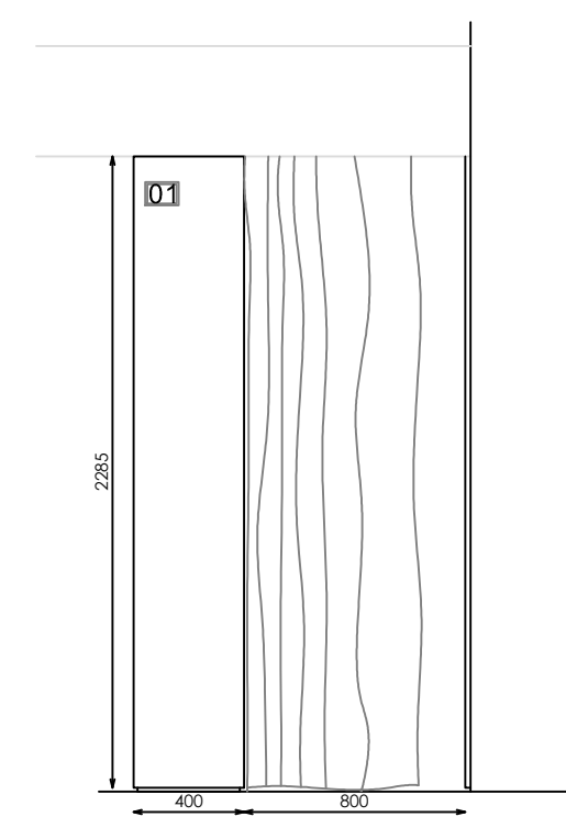
ALZADO
