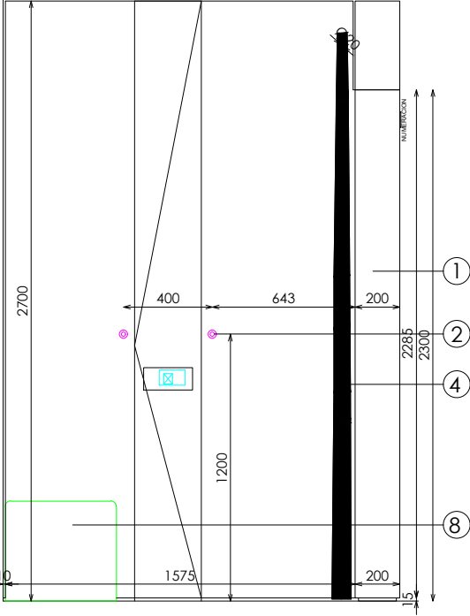
ALZADO LATERAL CUELGA
