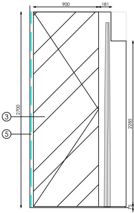
ALZADO LATERAL ESPEJO (C-C)
