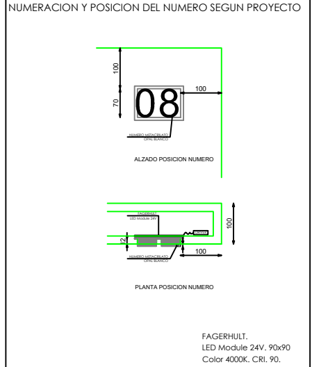
DETALLE NUMERO PROBADORES
