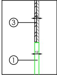
DETALLE A
