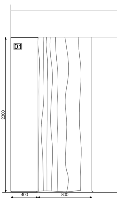
ALZADO
