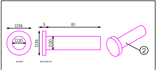
DETALLE A
