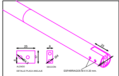
DETALLE CERRADURA ESPEJO/PANEL REGISTRABLE
