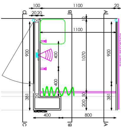
PLANTA
