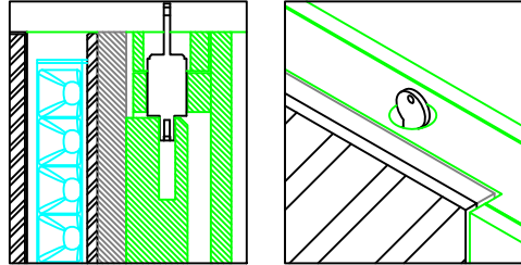
DETALLE CERRADURA ESPEJO/PANEL REGISTRABLE
