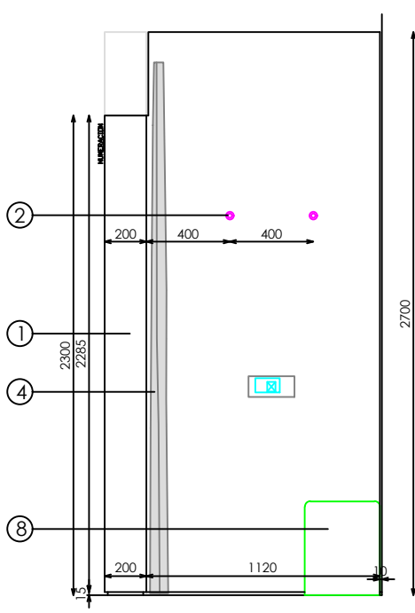
ALZADO LATERAL CUELGA (B-B)
