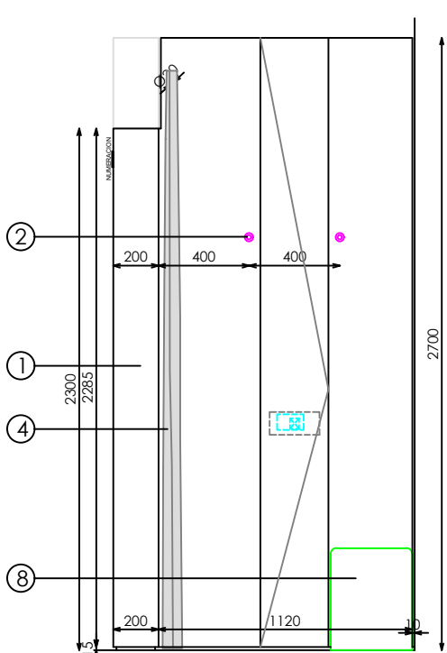
ALZADO LATERAL CUELGA (B-B)
