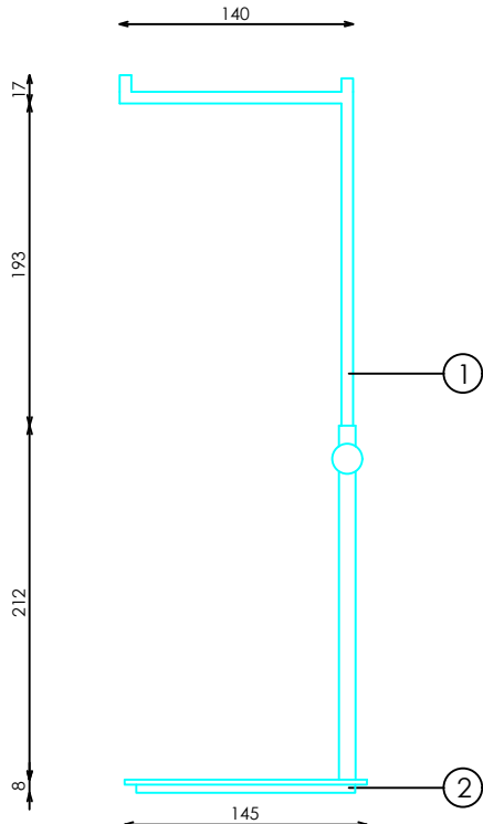
PERFIL
