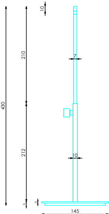
ALZADO
