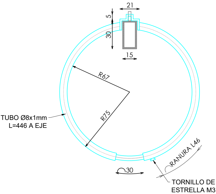
ALZADO
