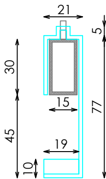
SECCIÓN
