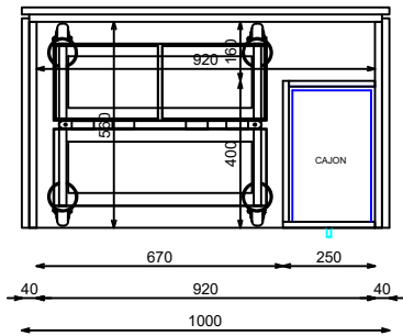
PLANTA SECCIONADA
