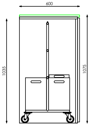
SECCION
