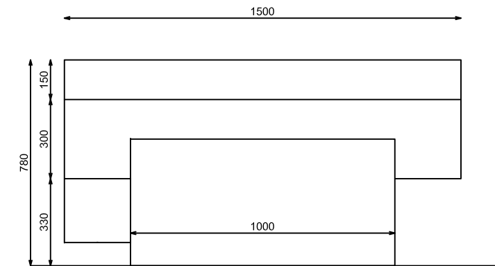
ALZADO LATERAL
