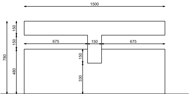
ALZADO FRONTAL
