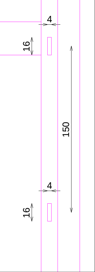
DETALLE D
