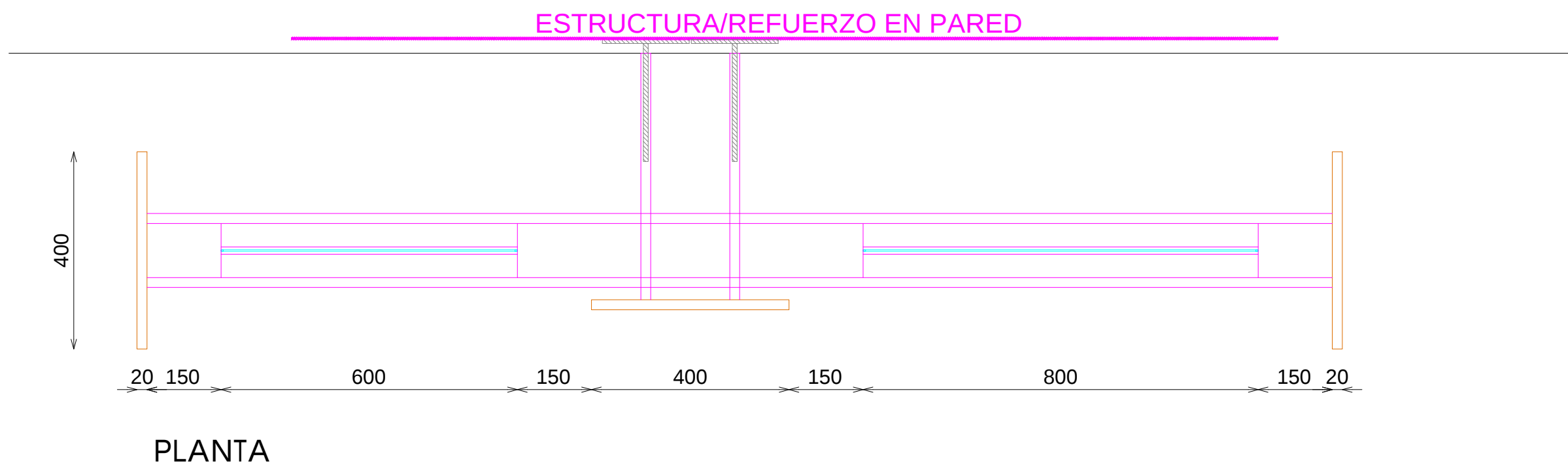
PLANTA
