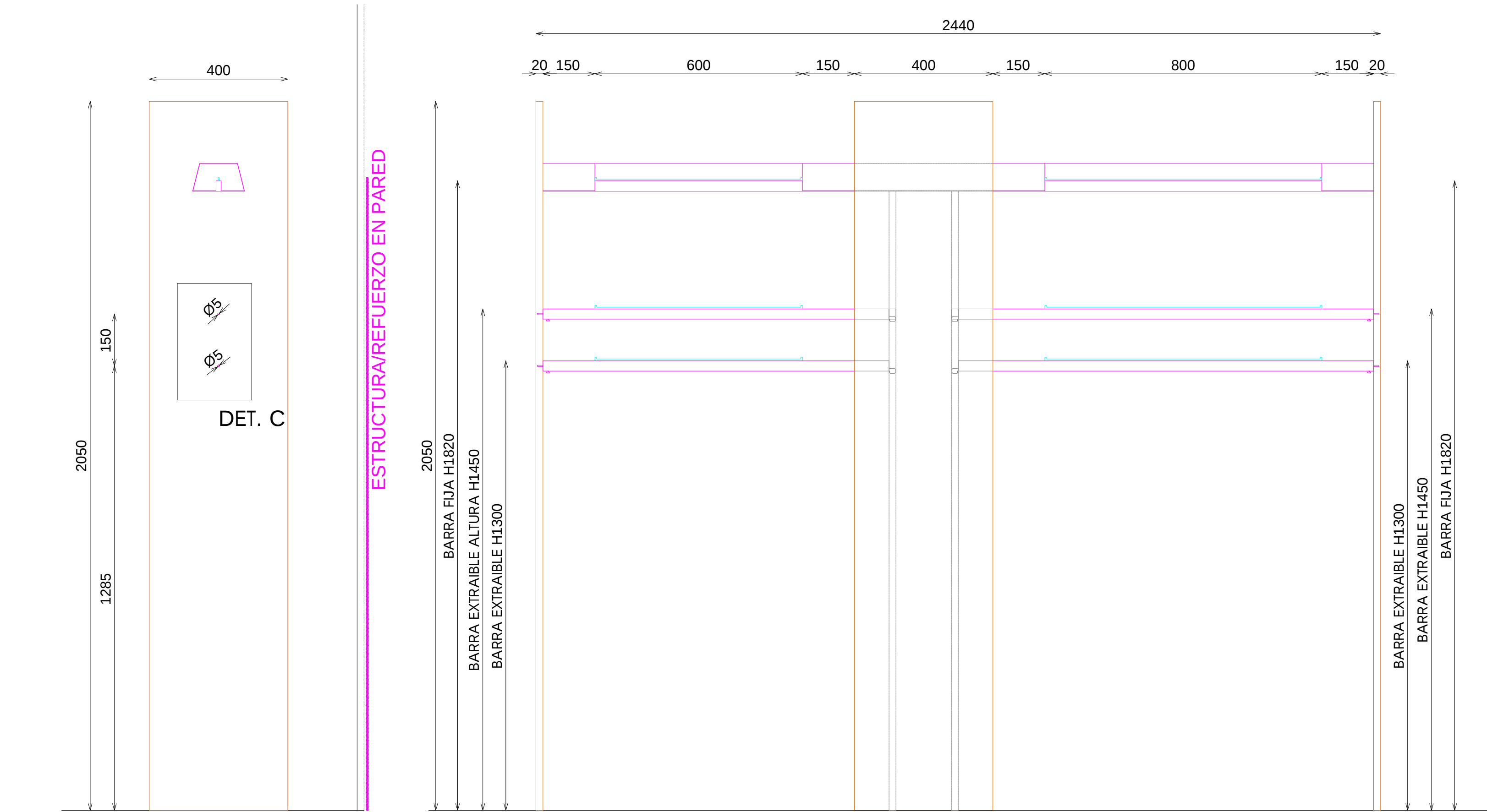
ALZADO (INTERIOR COSTADO IZQDO)
