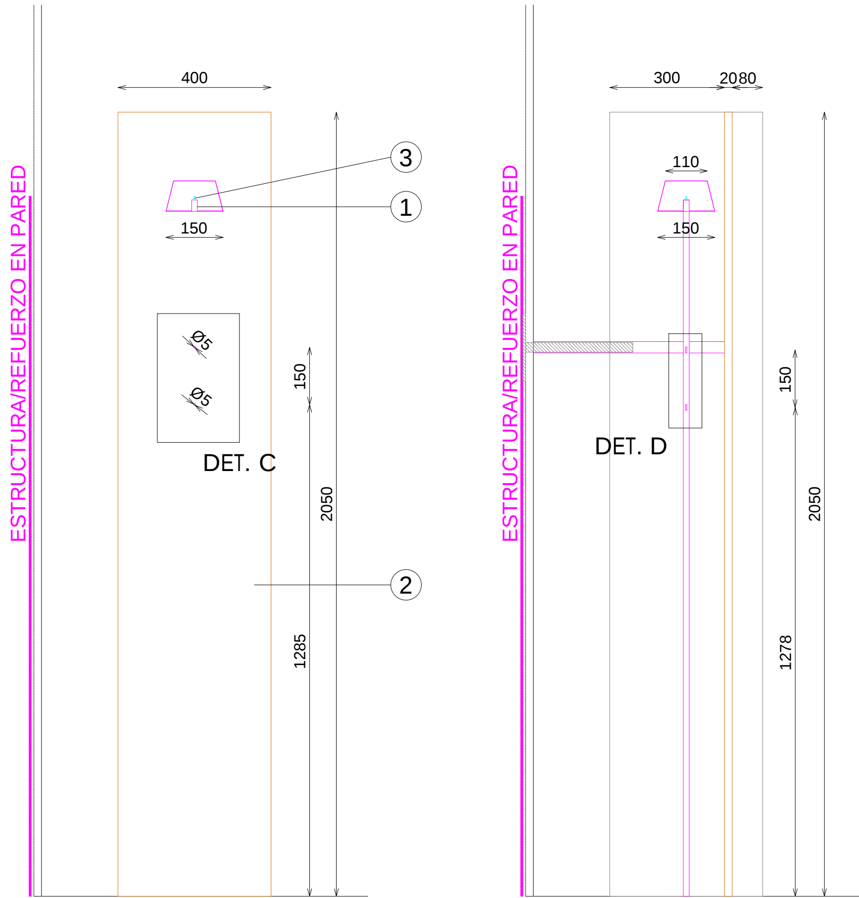
ALZADO (INTERIOR COSTADO DCHO)
