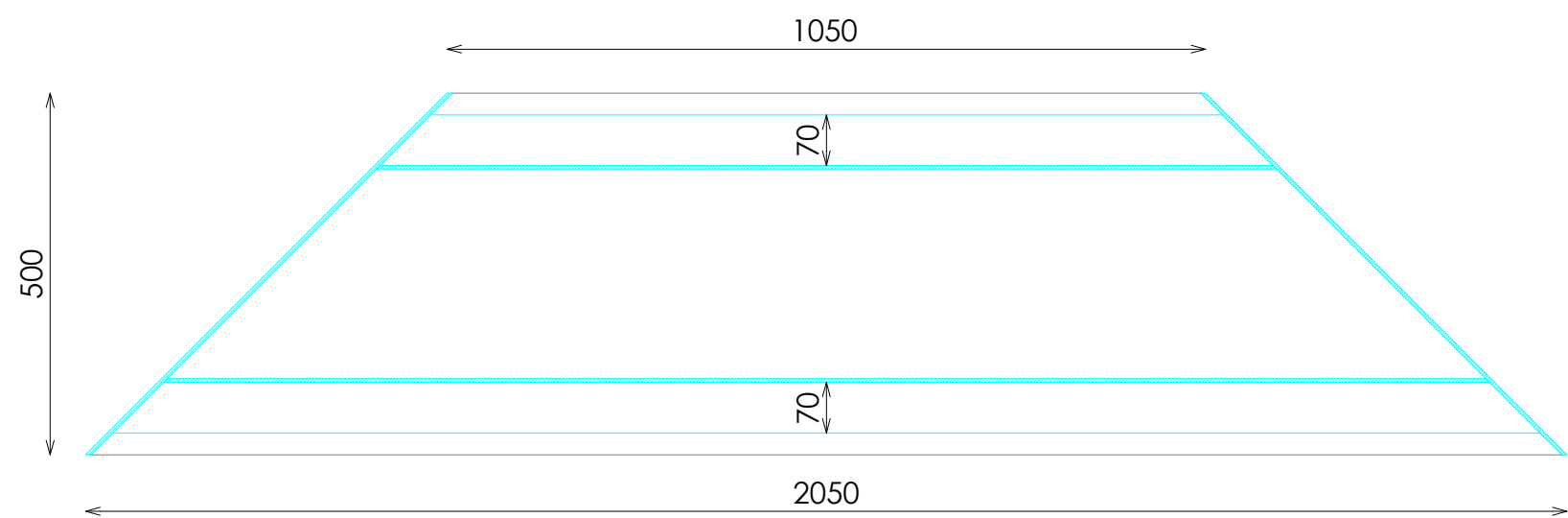
PLANTA SECCIONADA
