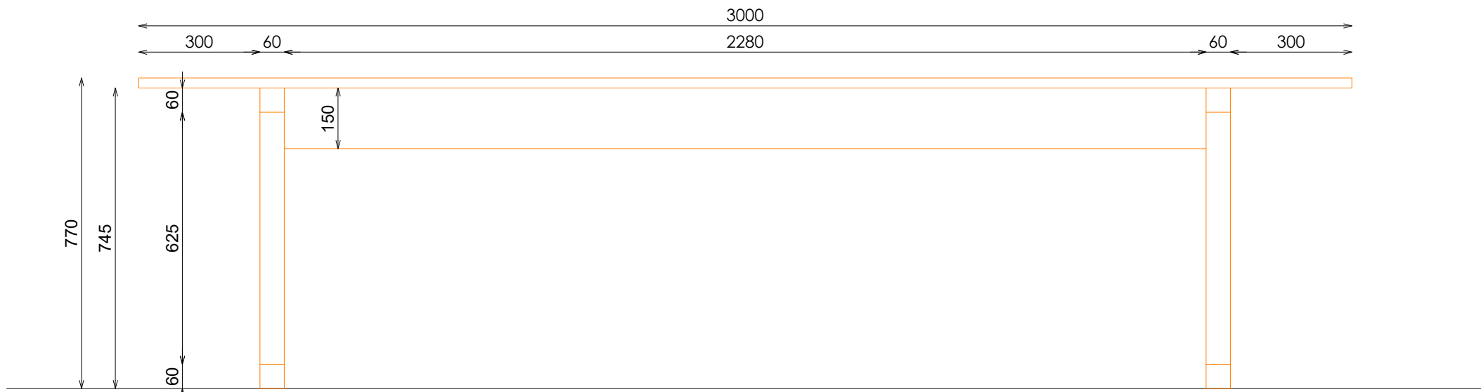
ALZADO FRONTAL
