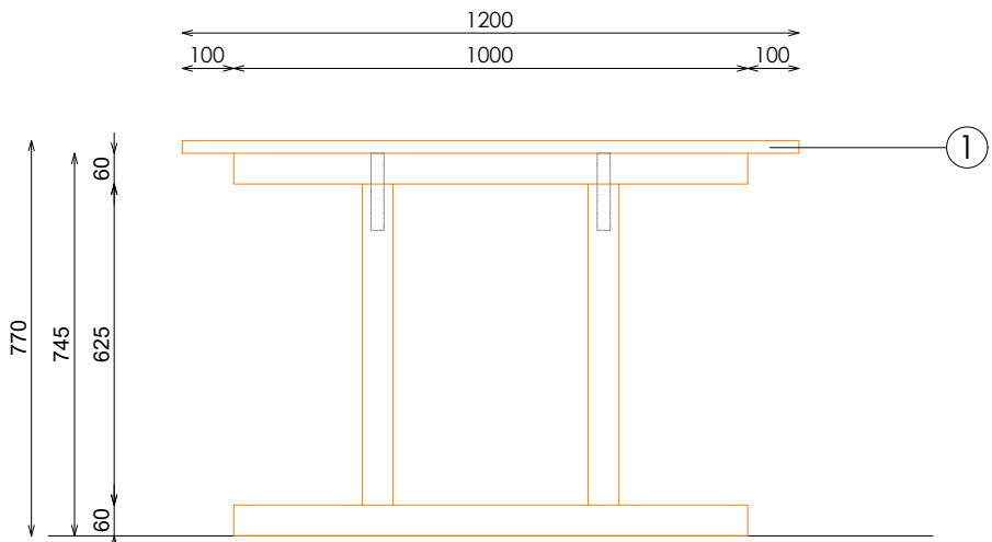
ALZADO LATERAL
