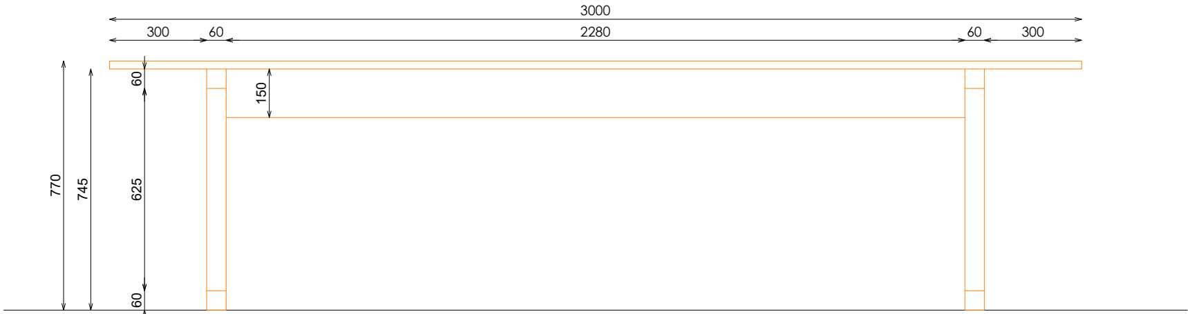
ALZADO FRONTAL
