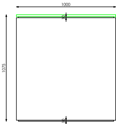
ALZADO FRONTAL
