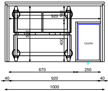
PLANTA SECCIONADA
