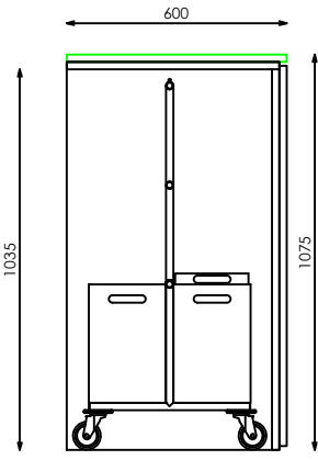
SECCION
