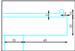
DETALLE B
