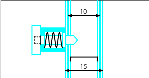
DETALLE SISTEMA ANCLAJE
