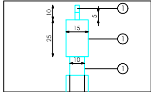
DETALLE B
