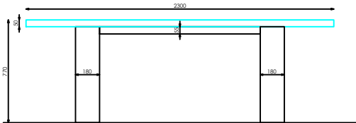
ALZADO FRONTAL
