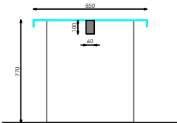
SECCION LATERAL
