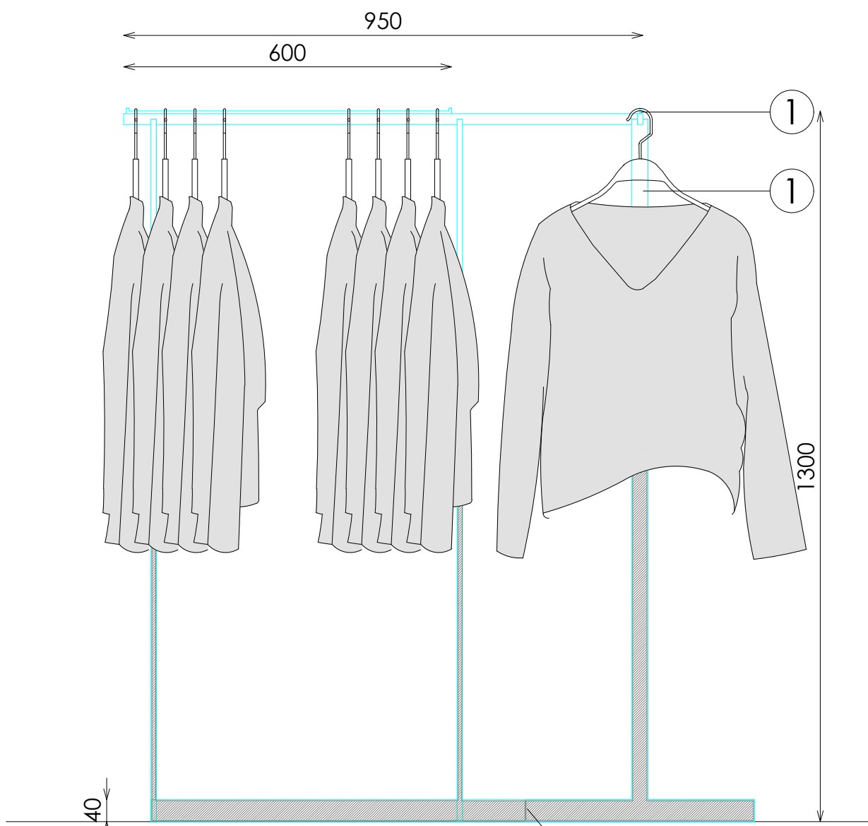
ALZADO LATERAL
