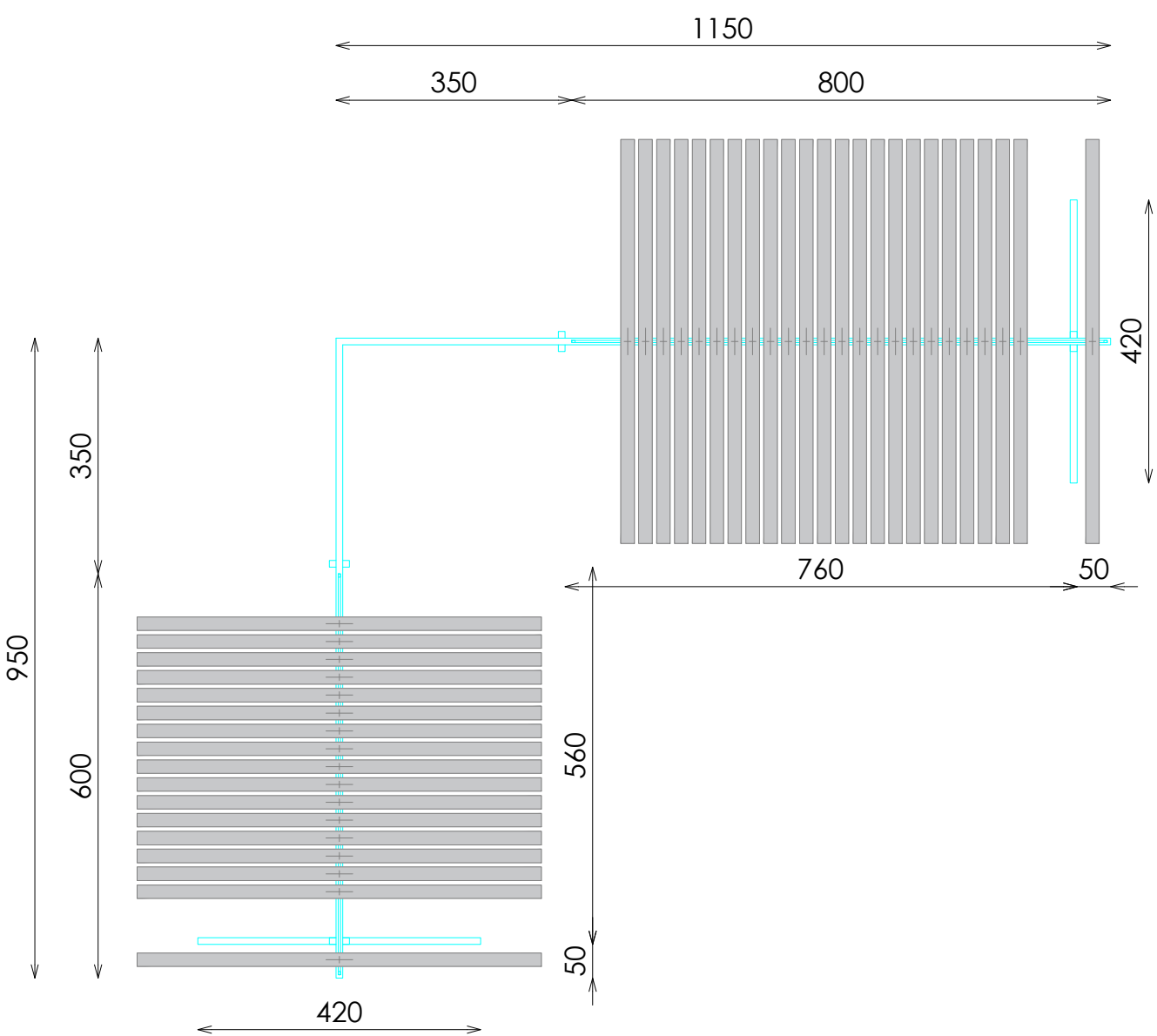
PLANTA
