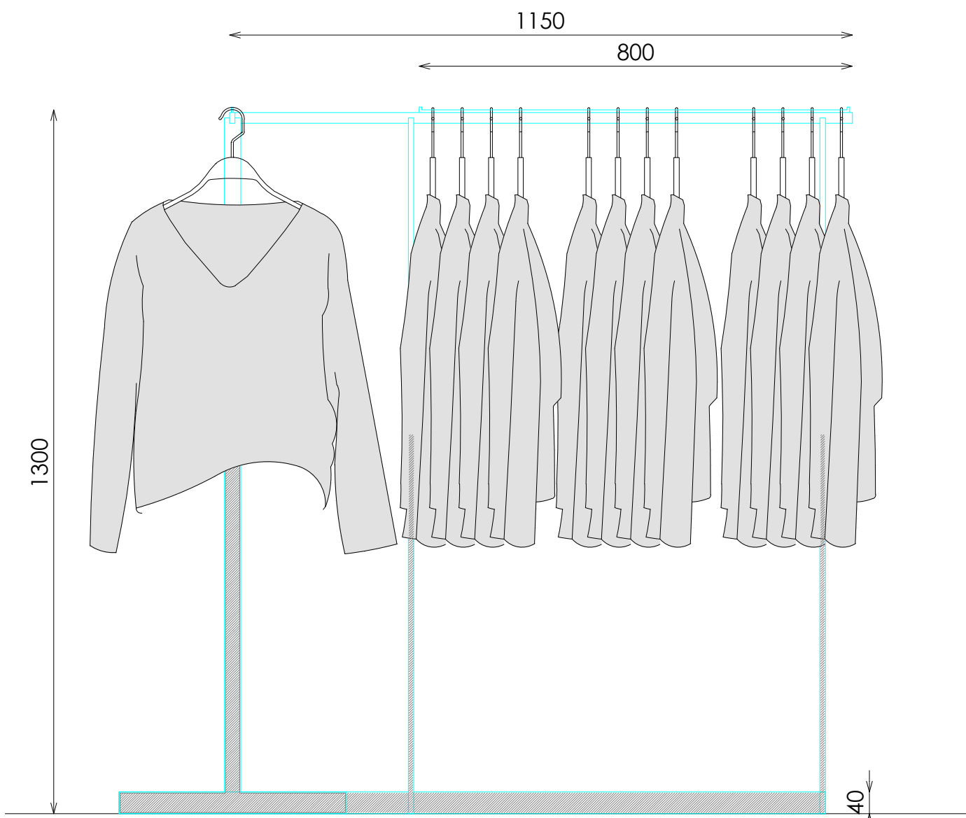
ALZADO FRONTAL
