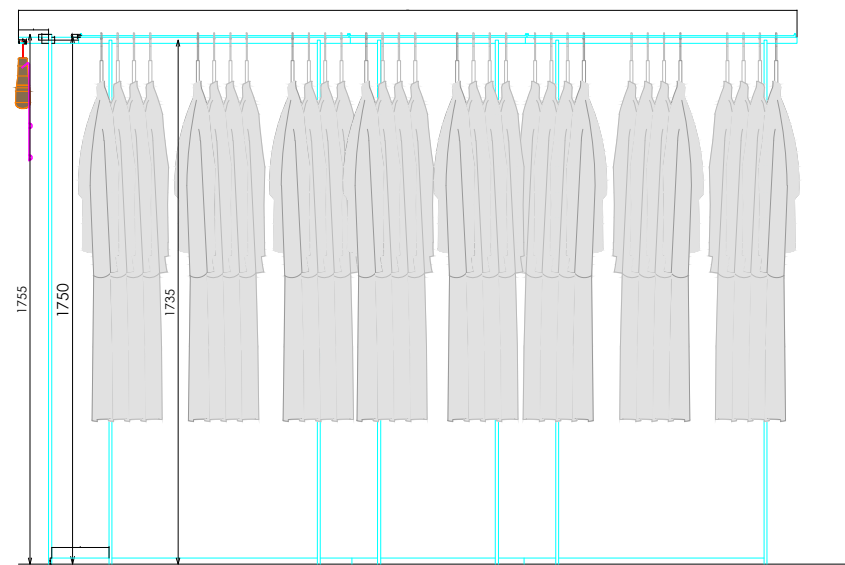
ALZADO FRONTAL
