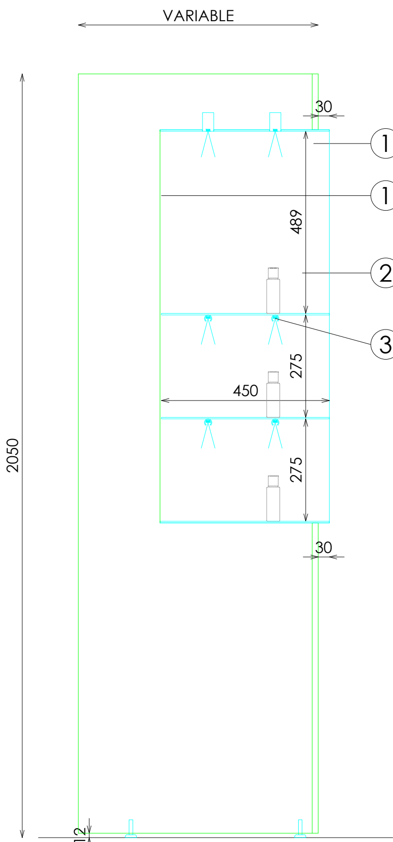
SECCIÓN TRANSVERSAL
