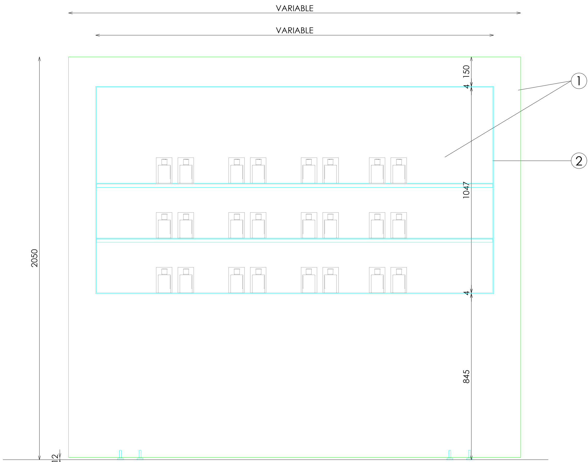
ALZADO FRONTAL
