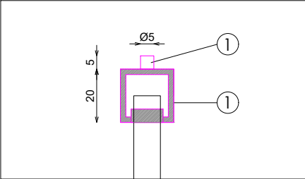
DETALLE TUBO SUPERIOR
