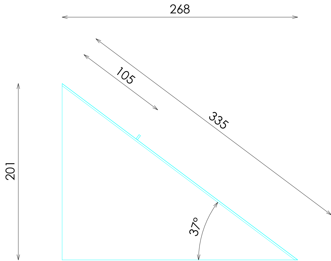
SECCIÓN
