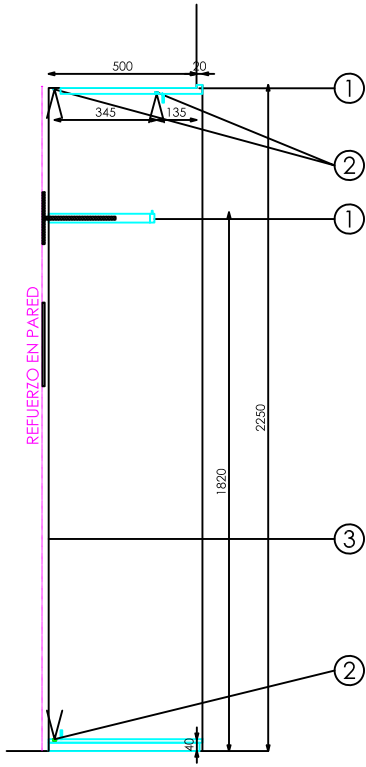
SECCIÓN
