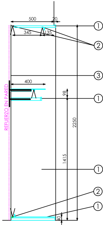
SECCIÓN
