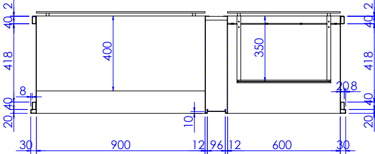
剖面 AI-AI
