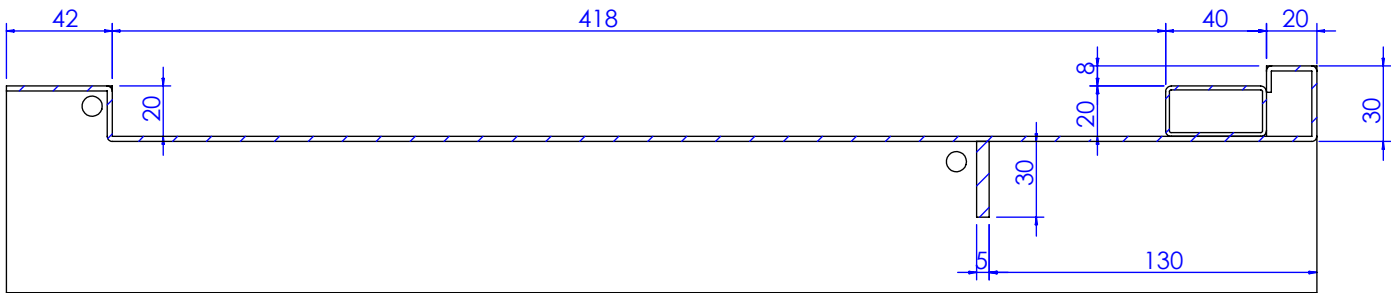
剖面 AG-AG
