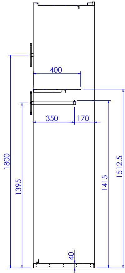
剖面 AG-AG
