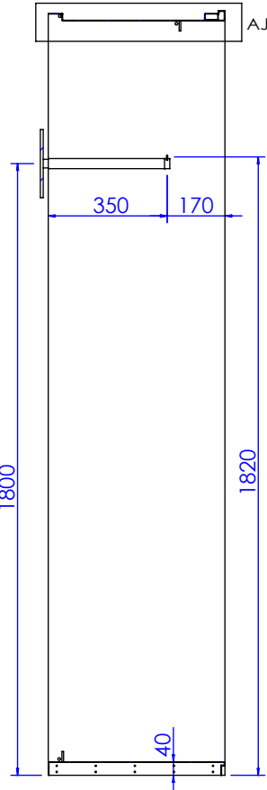
剖面 AH-AH
