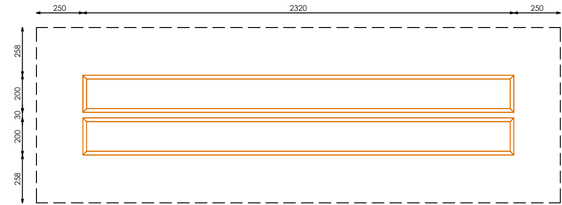
PLANTA (SECCION PATAS)
