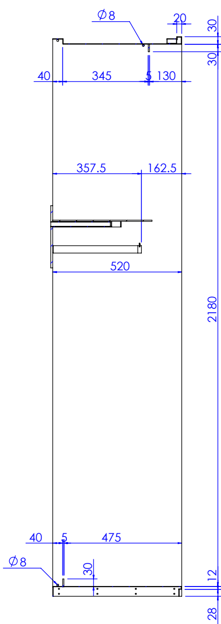
剖面 AG-AG
