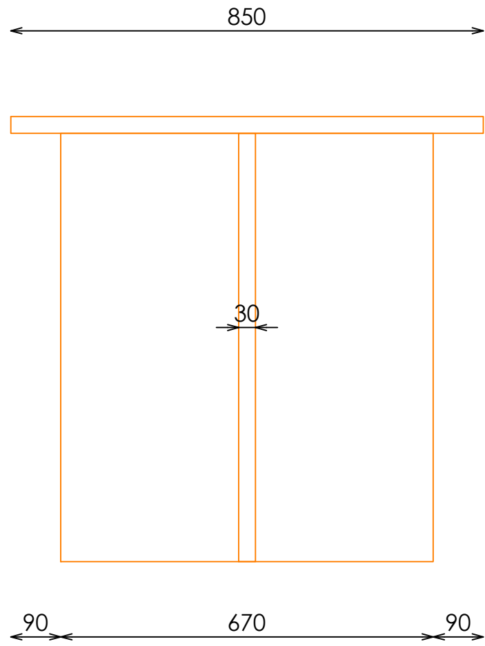
ALZADO IZQUIERDA
