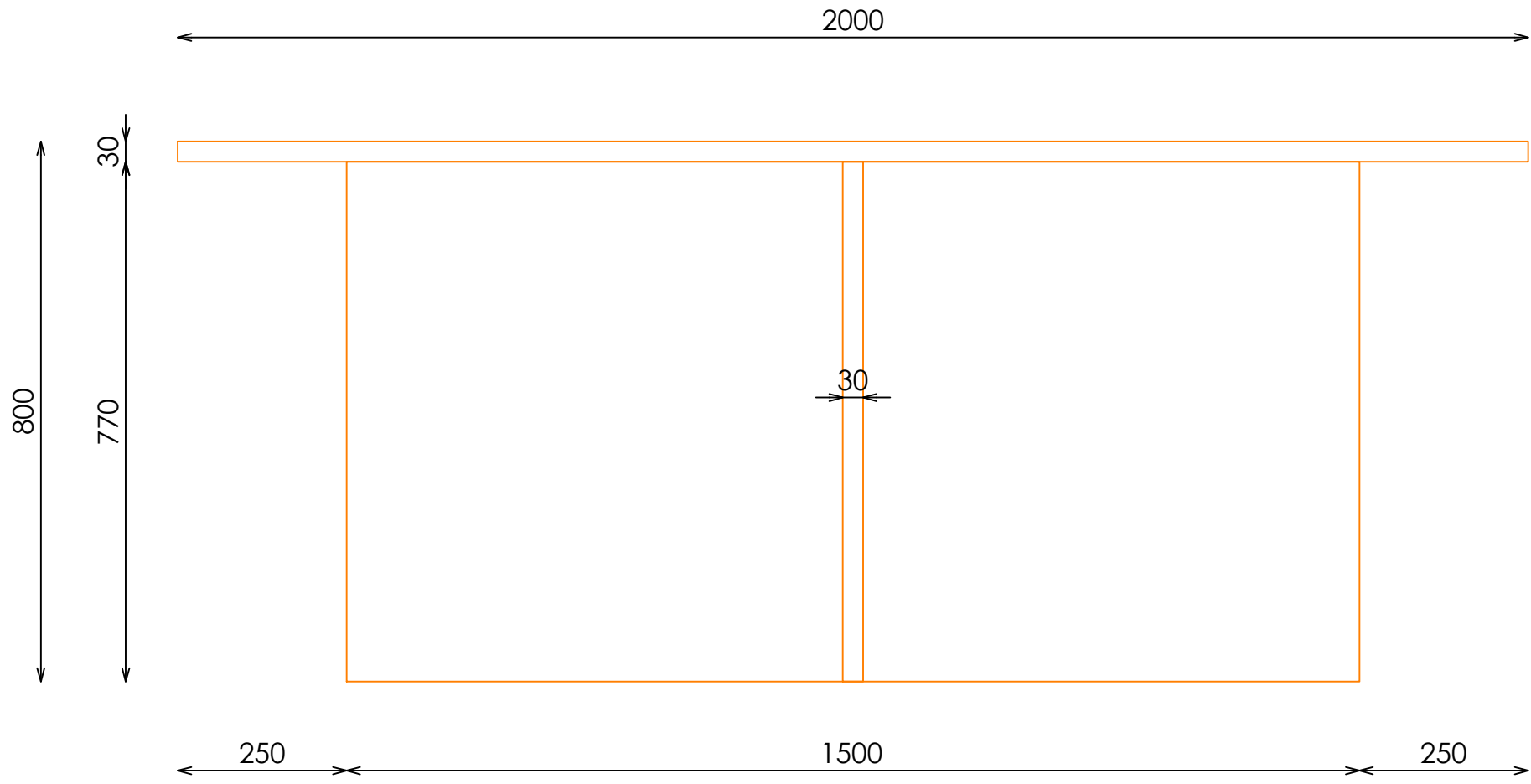
ALZADO FRONTAL
