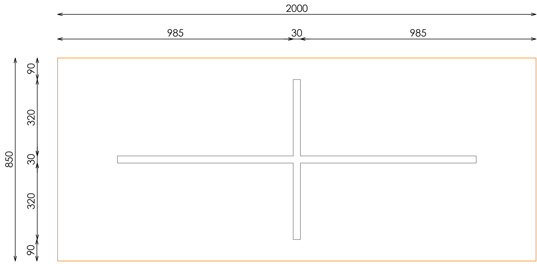
PLANTA
