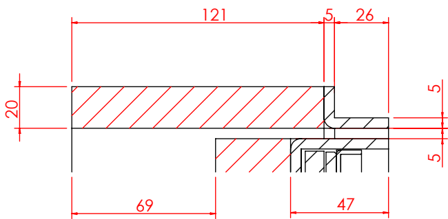
局部视图 AI 比例 2 : 5
