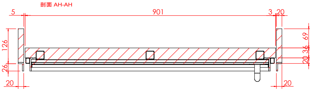
剖面 AJ-AJ 比例 1 : 8
